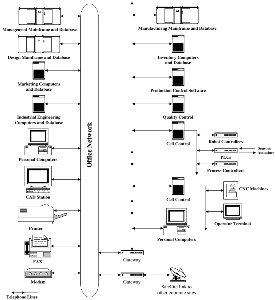
รูปที่ 1.1: ระบบ CIM
